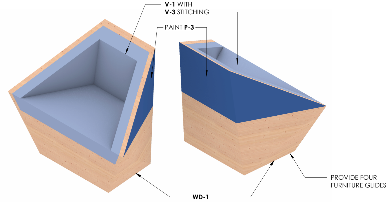
3 TEEN TAG CHAIR AXONOMETRIC A842
