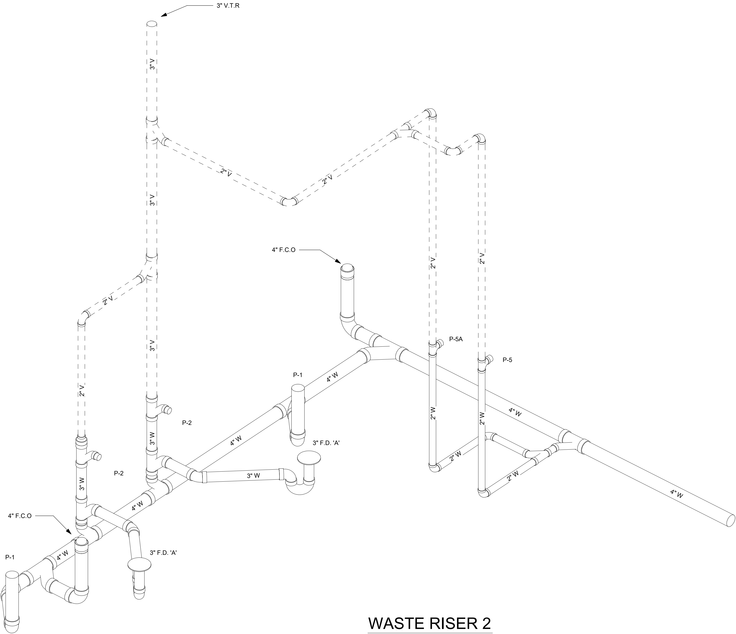
WASTE RISER 2 SCALE: N.T.S.
