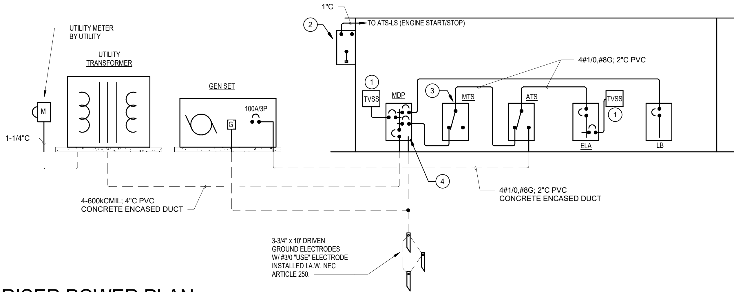
RISER POWER PLAN SCALE: 12" = 1'-0"
