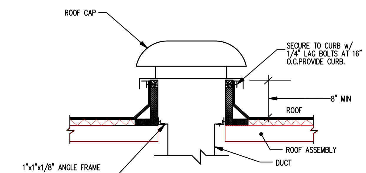
4 ROOF CAP DETAIL SCALE: N.T.S.
