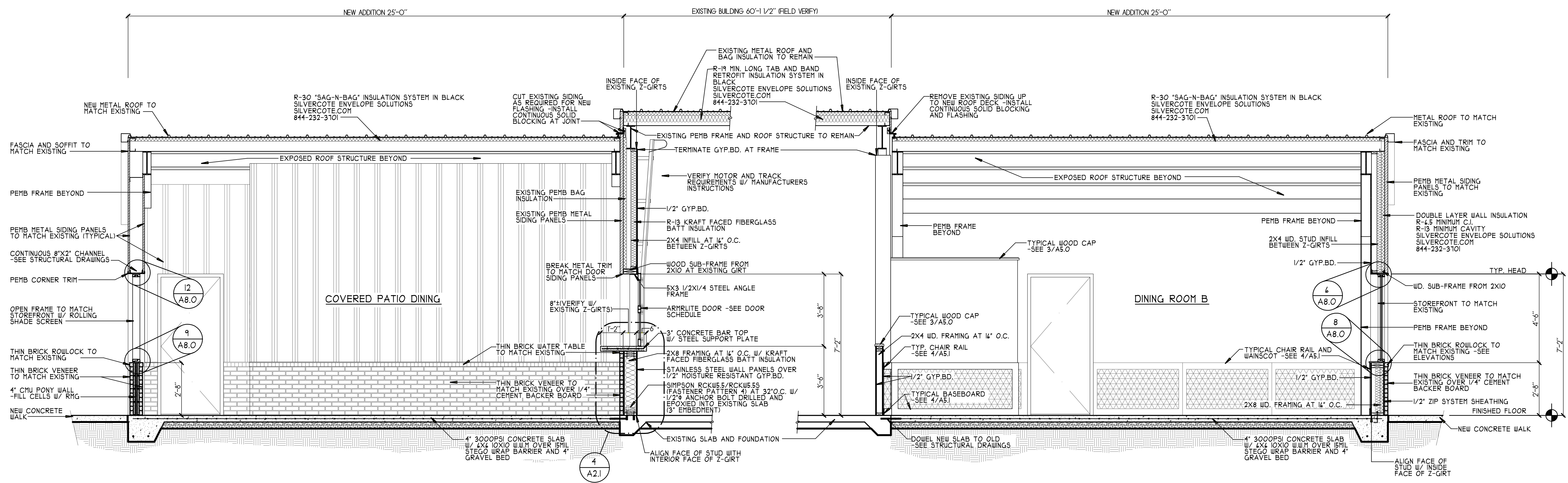
PARTIAL SECTION SCALE: 3/8" = 1'-0"
