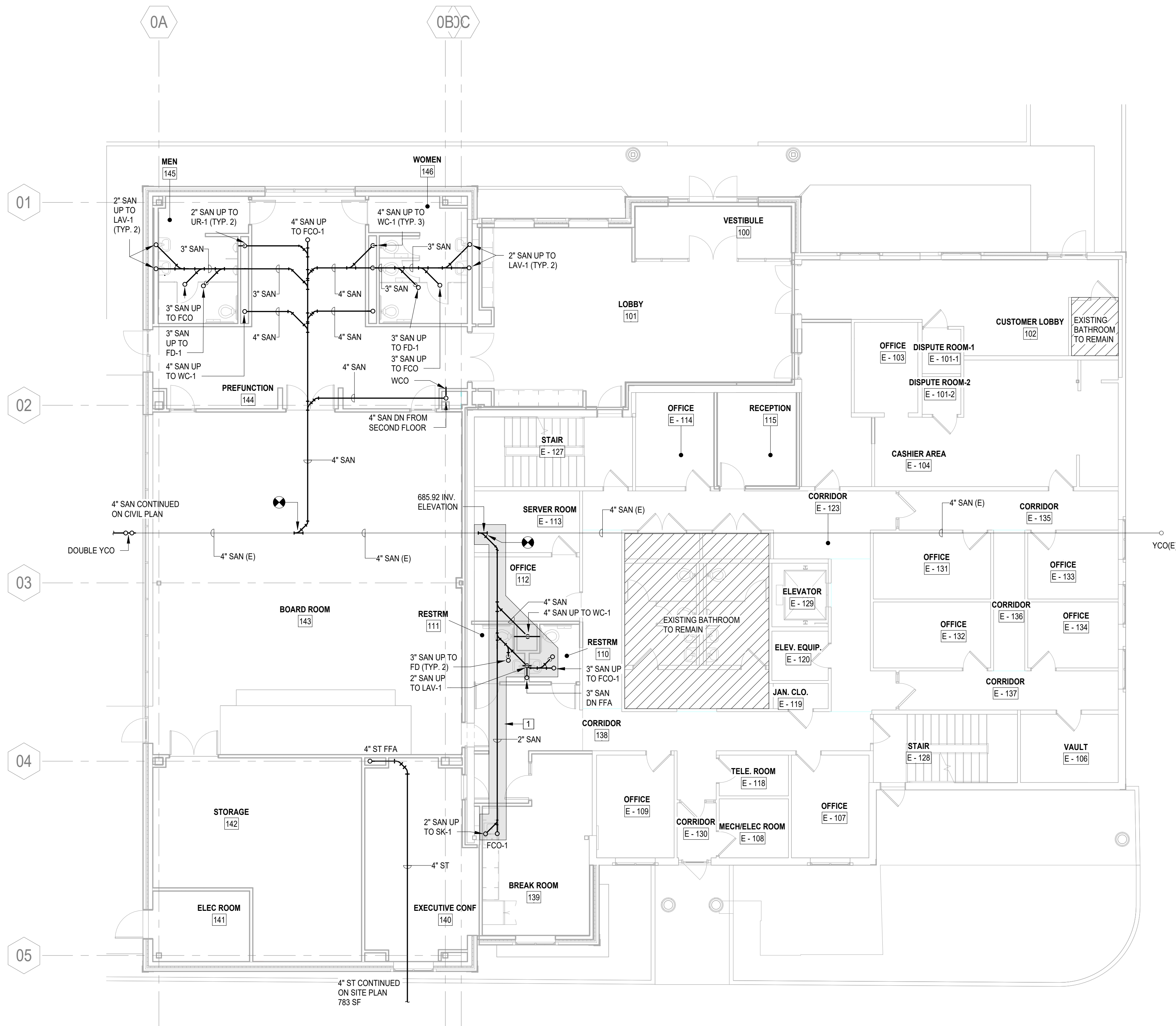
1 BELOW GRADE PLAN SCALE: 1/8" = 1'-0"
