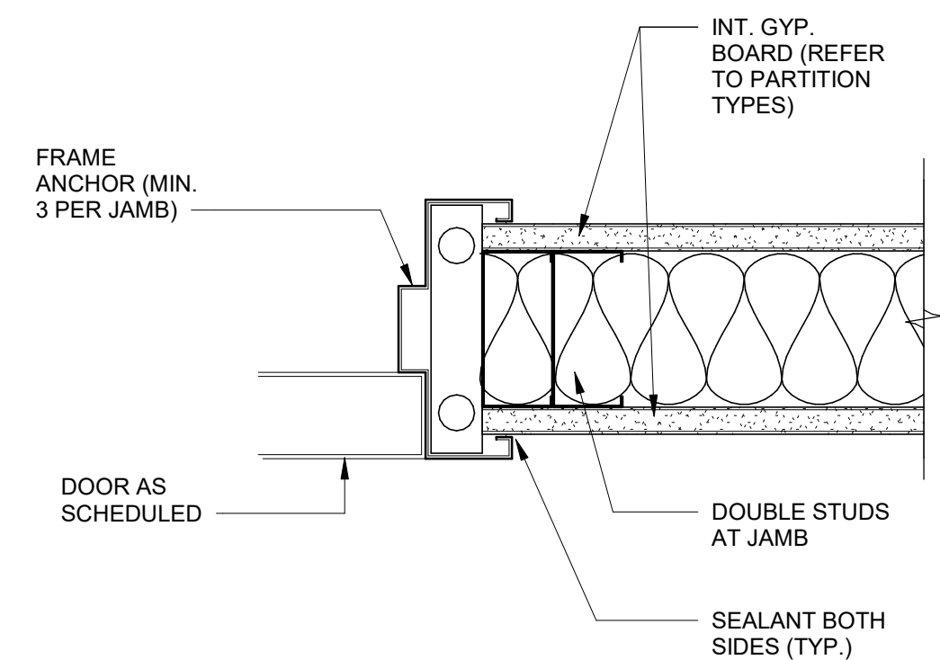
9 HM TYP. JAMB A-802 | 3" = 1'-0"
