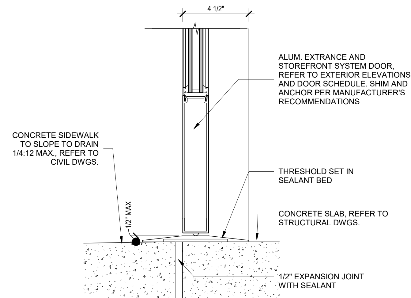
14 SILL STOREFRONT DR A-802 | 3" = 1'-0"
