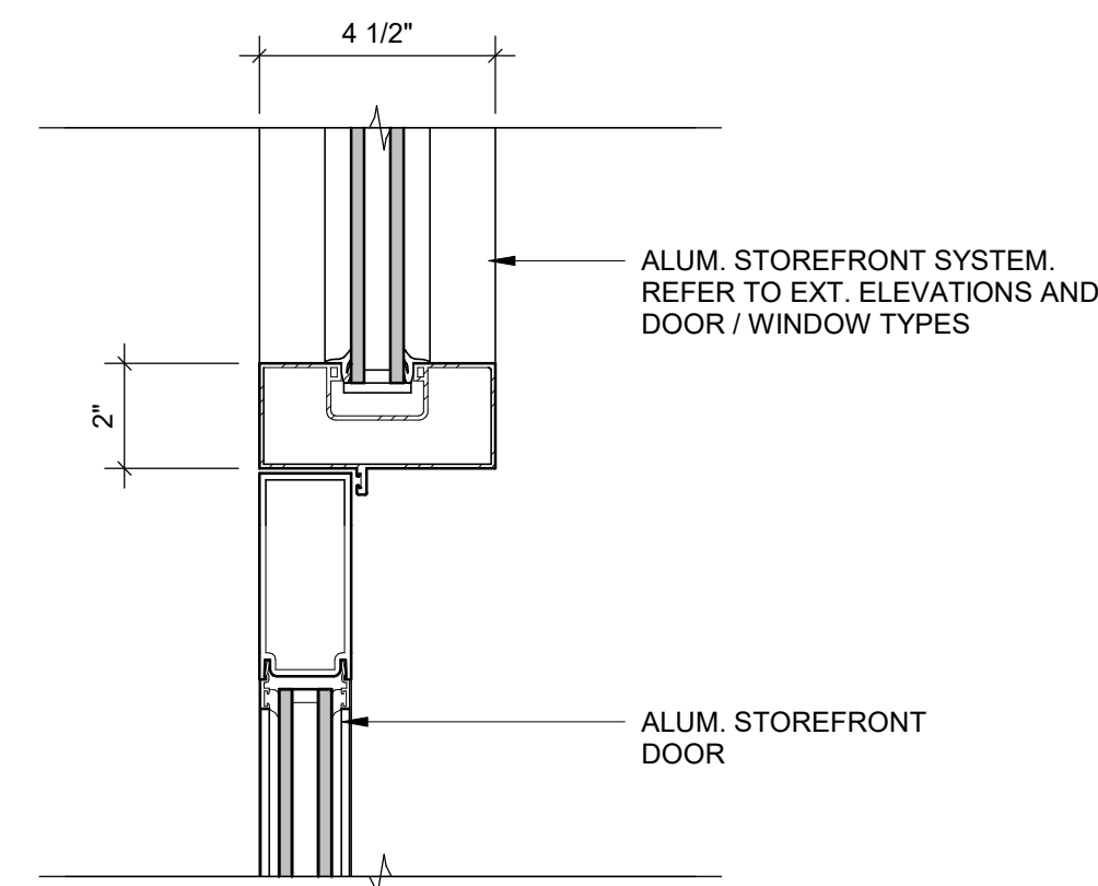
3 STOREFRONT HEAD A-802 | 3" = 1'-0"
