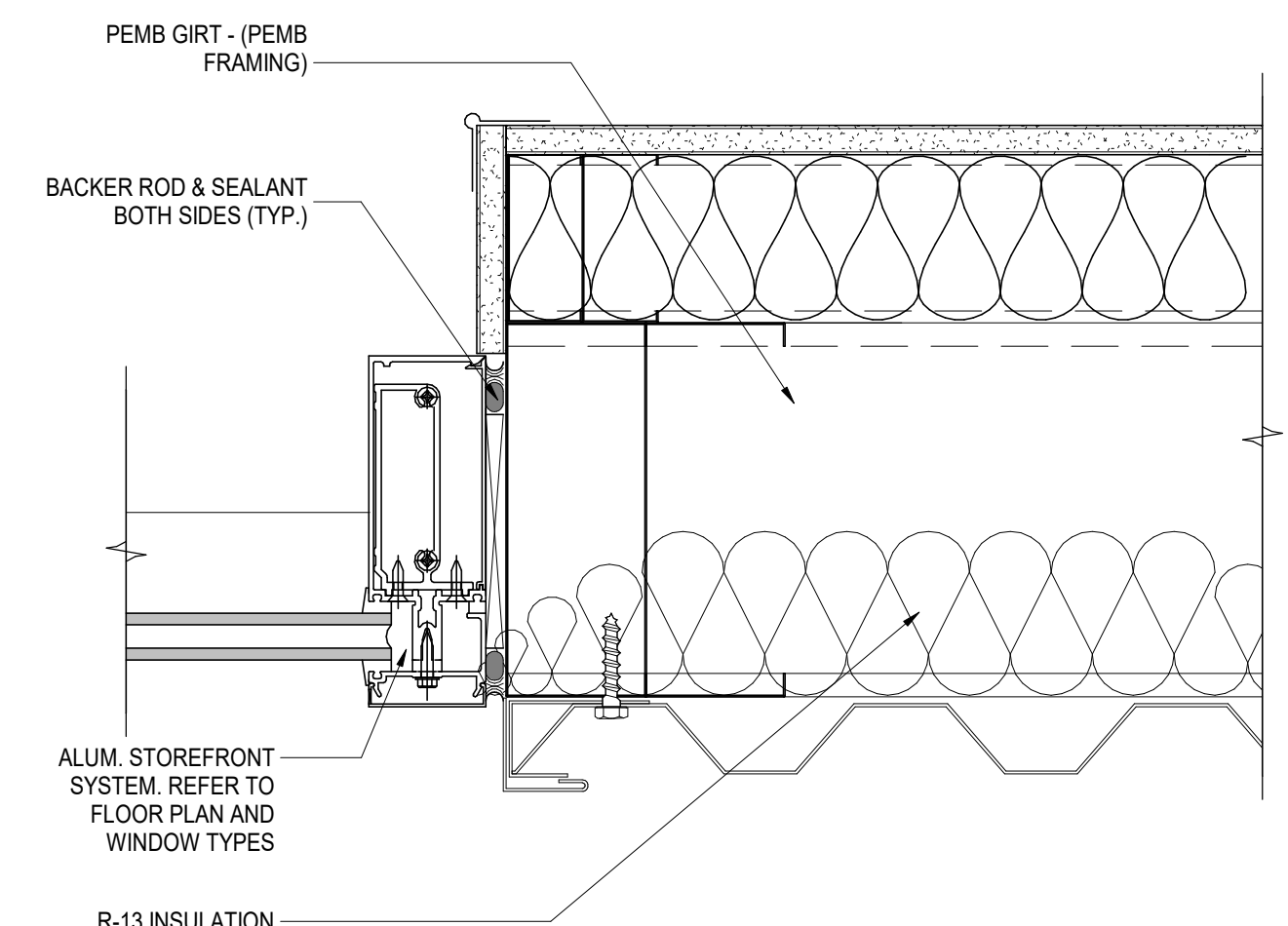
16 STOREFRONT / WINDOW JAMB - PEMB A-802 | 3" = 1'-0"
