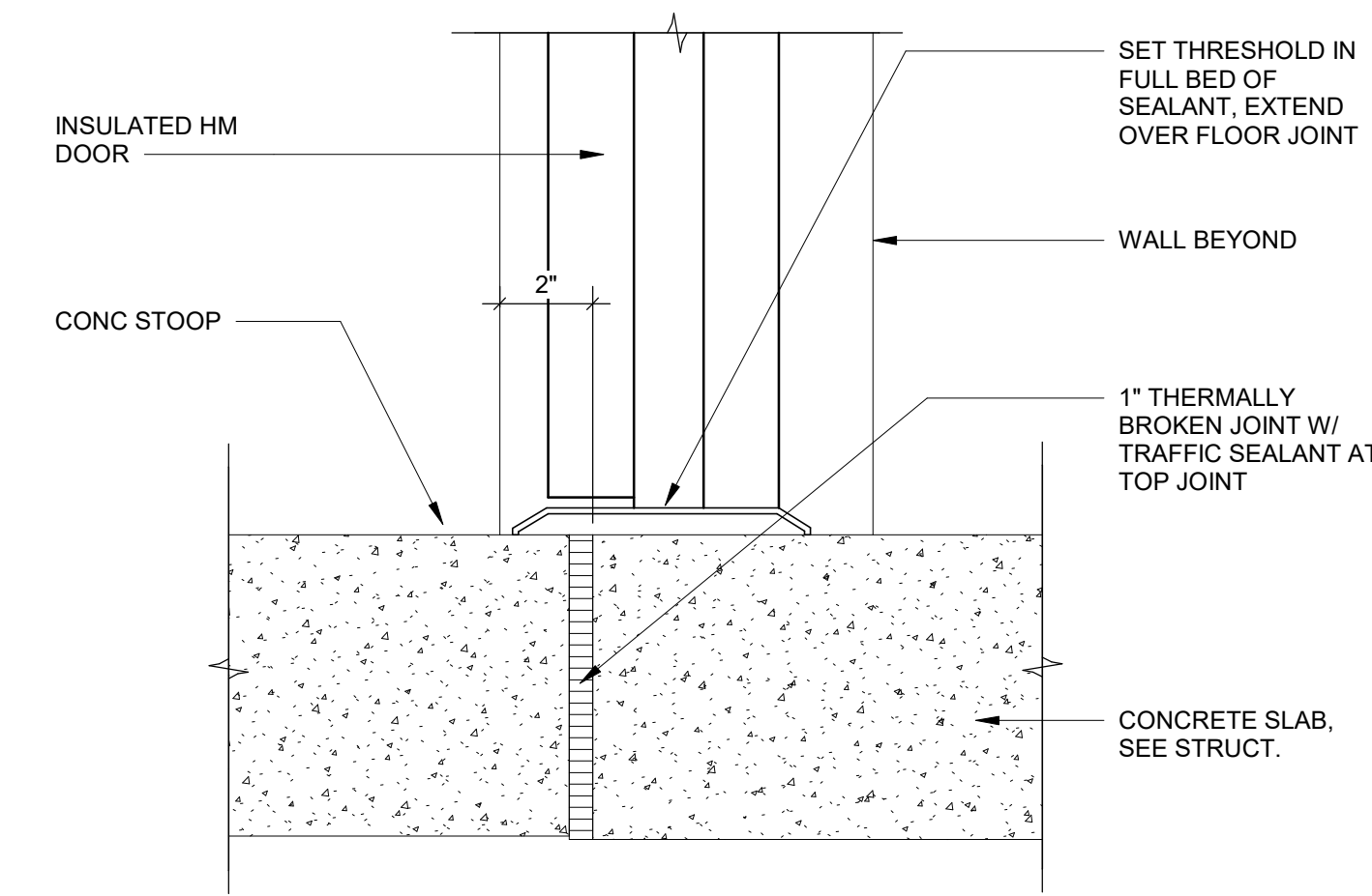
15 HM DOOR SILL A-802 | 3" = 1'-0"
