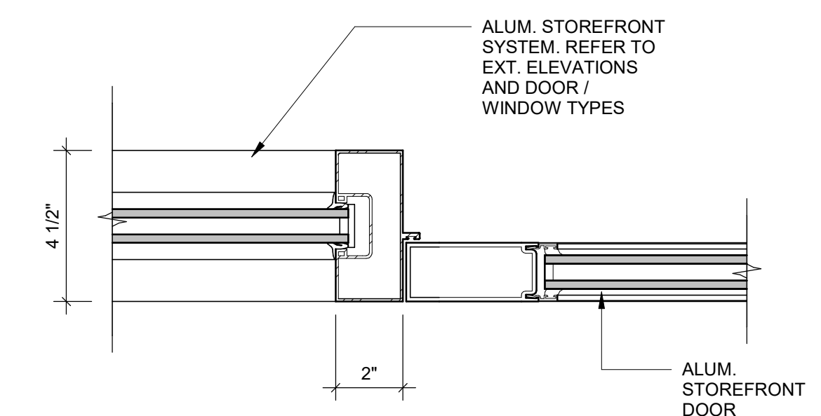
12 STOREFRONT JAMB A-802 | 3" = 1'-0"
