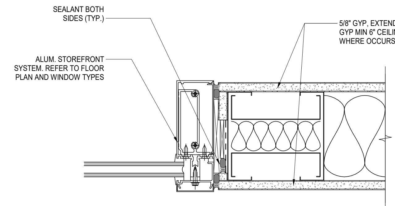
11 STOREFRONT / WINDOW JAMB - GYP A-802 | 3" = 1'-0"
