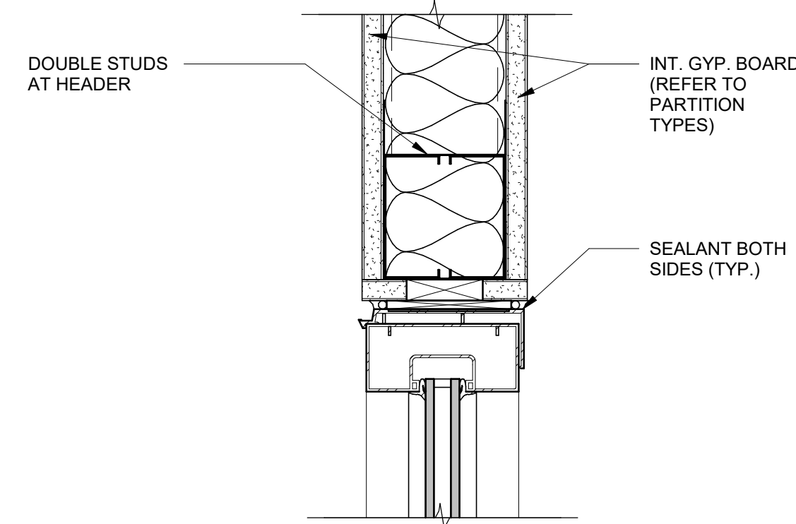
6 ALUM. STOREFRONT INT. HEAD A-802 | 3" = 1'-0"
