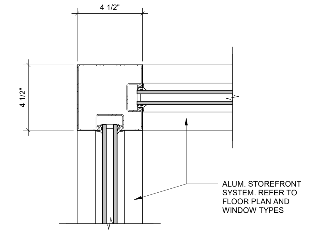
8 CORNER STOREFRONT A-802 | 3" = 1'-0"
