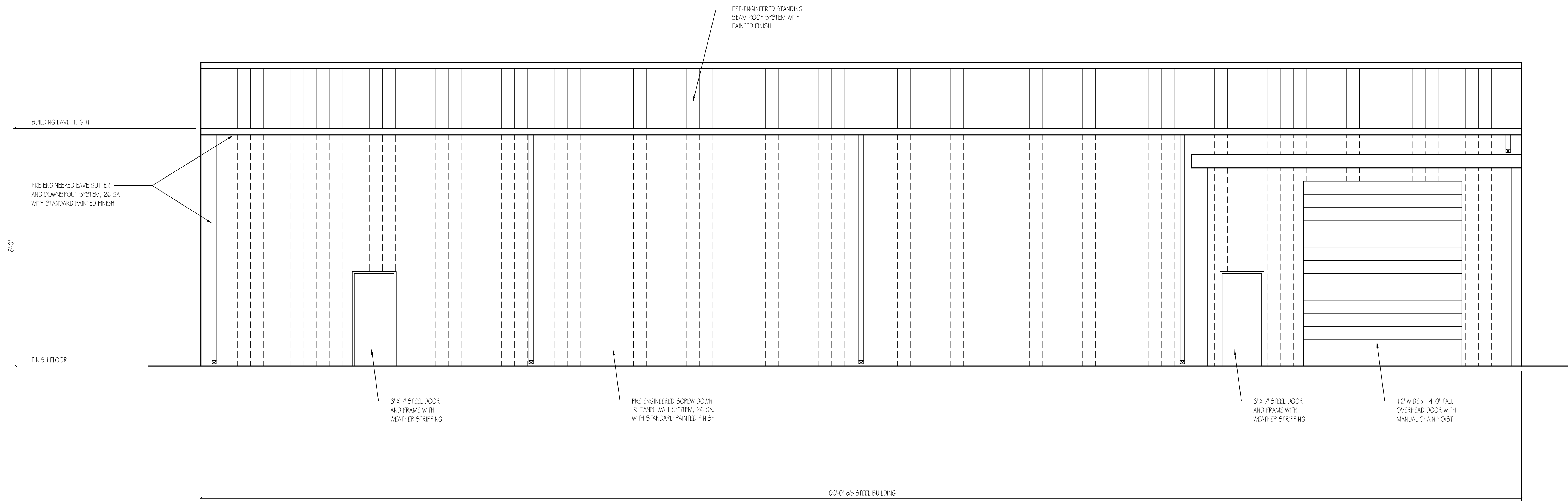
Elevation SCALE: 1/4" = 1'-0"
