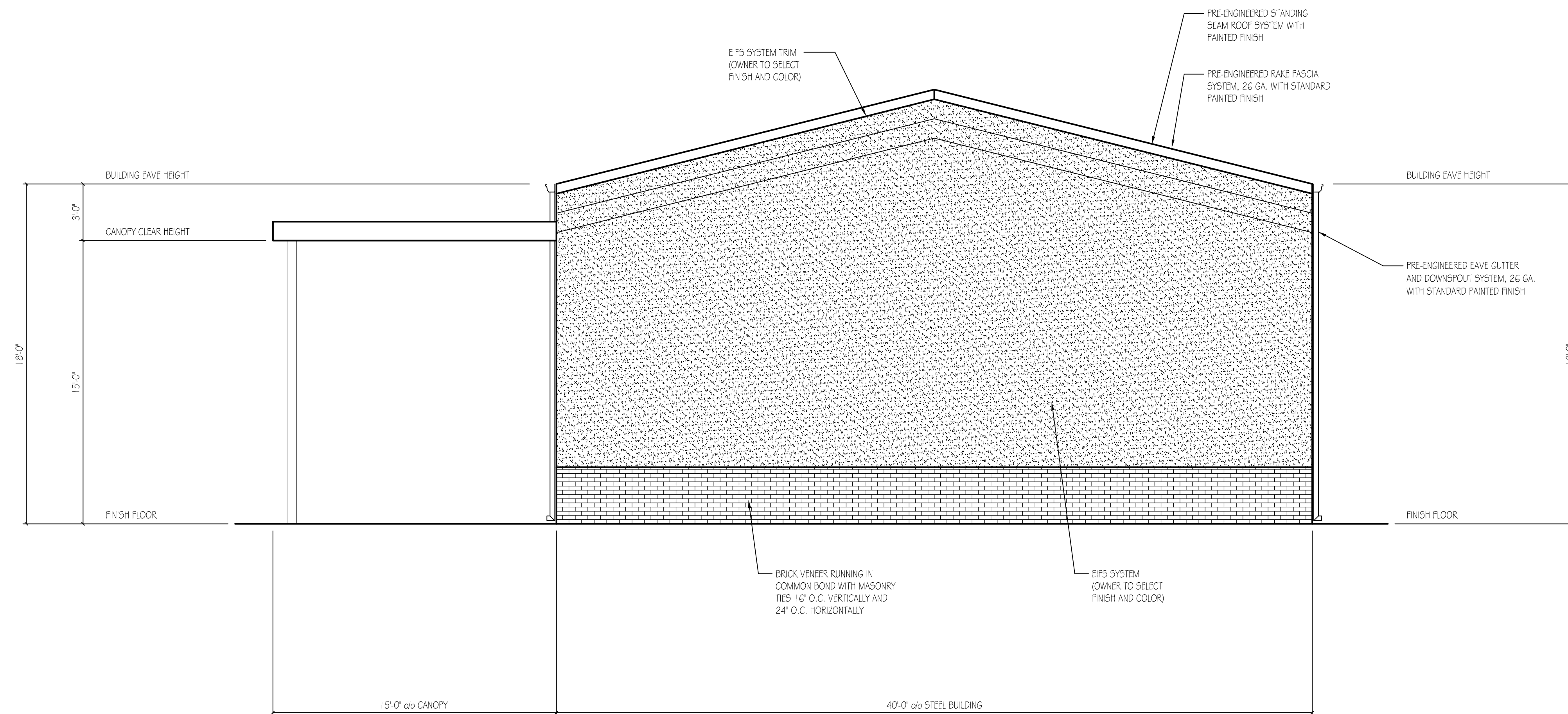
Elevation SCALE: 1/4" = 1'-0"
