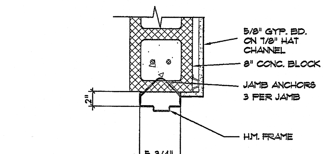
14 DOOR JAMB DETAIL SCALE: 1 1/2\"/>
