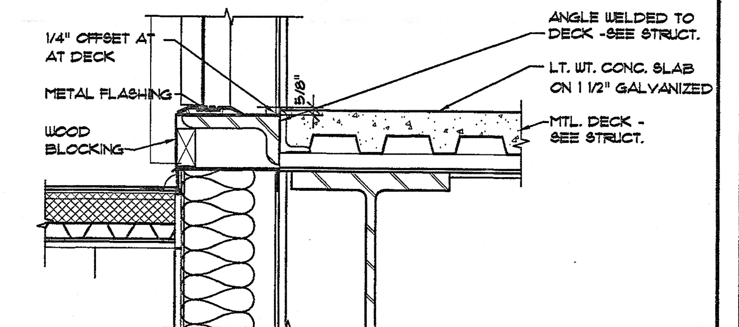
25 DOOR SILL SECTION SCALE: 1 1/2\"/>
