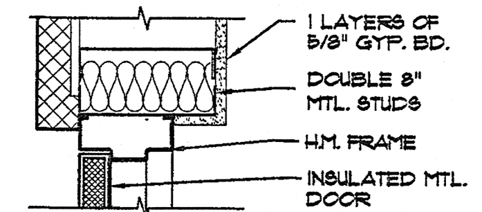
24 DOOR JAMB DETAIL SCALE: 1 1/2\"/>
