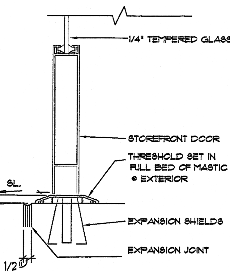
5 DOOR SILL DETAIL SCALE: 3\"/>
