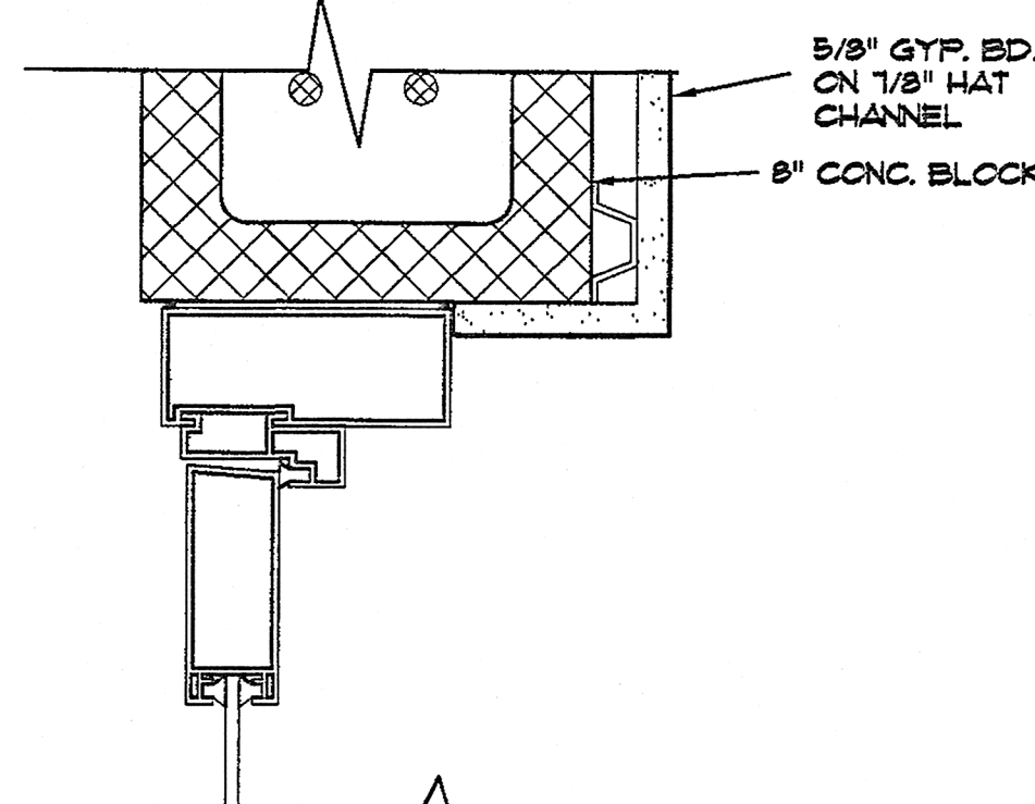
4 DOOR JAMB DETAIL SCALE: 3\"/>
