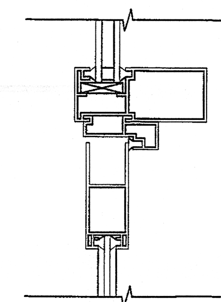
2 DOOR HEAD DETAIL SCALE: 3\"/>
