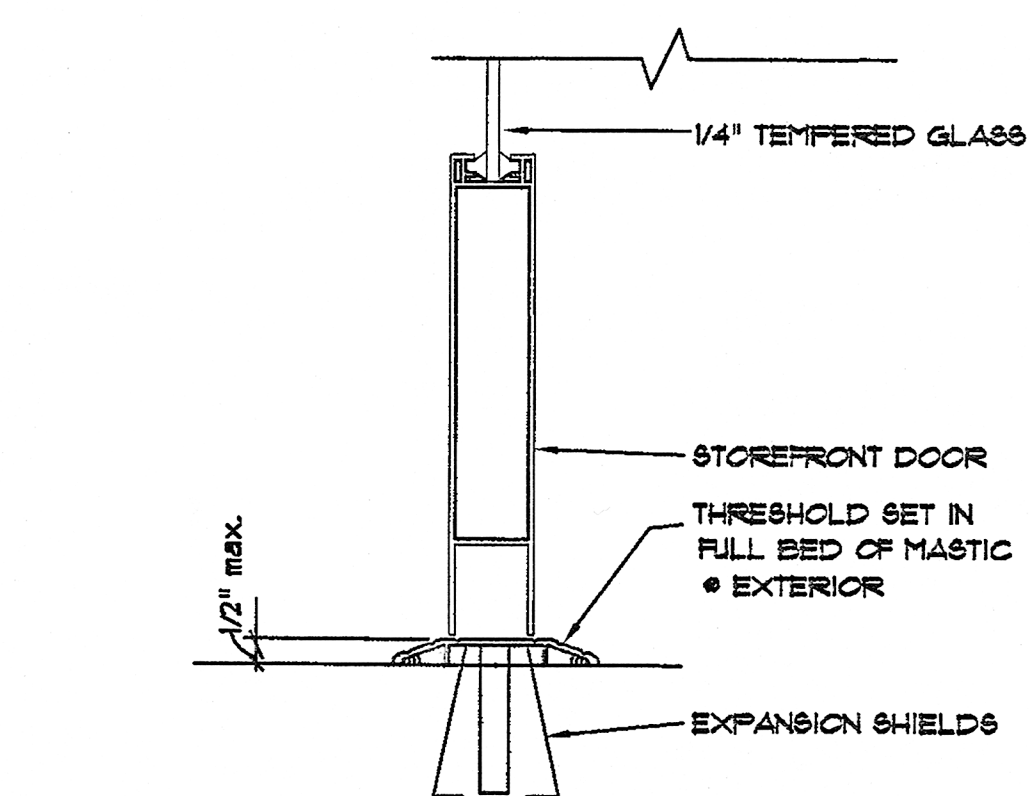
10 DOOR SILL DETAIL SCALE: 3\"/>
