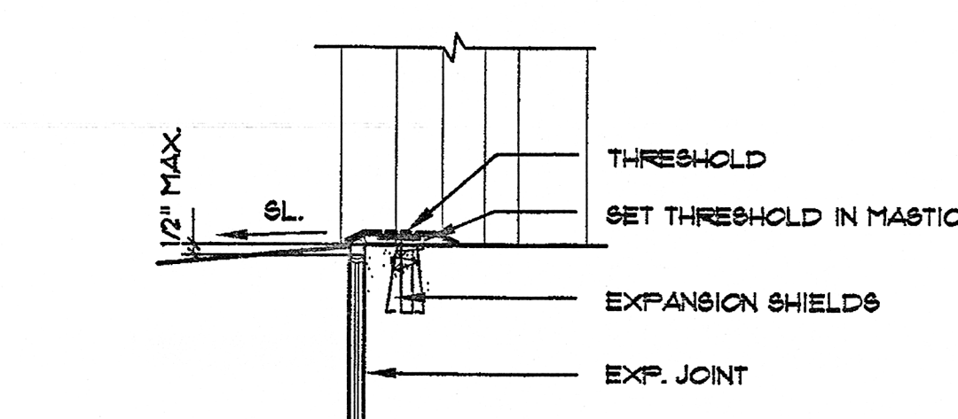
16 DOOR SILL SECTION SCALE: 1 1/2\"/>
