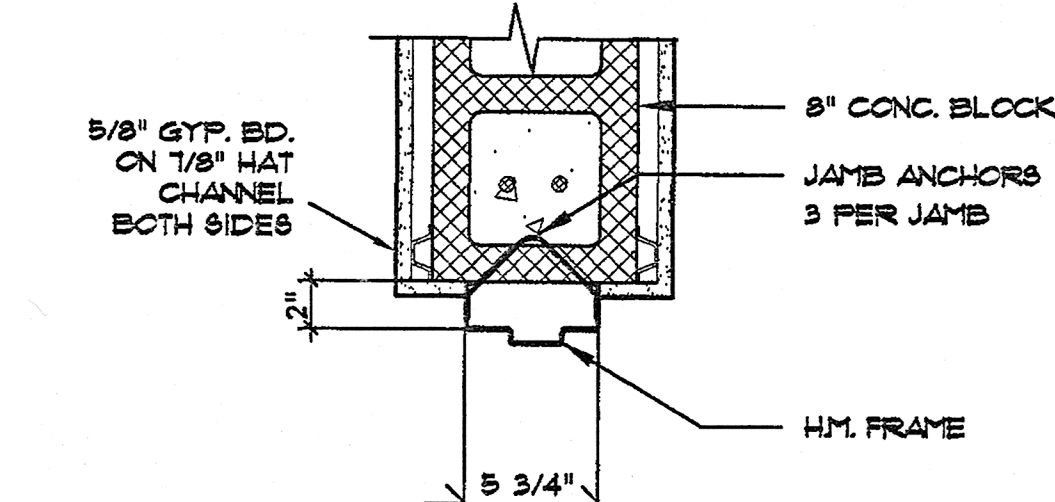
13 DOOR JAMB DETAIL SCALE: 1 1/2\"/>
