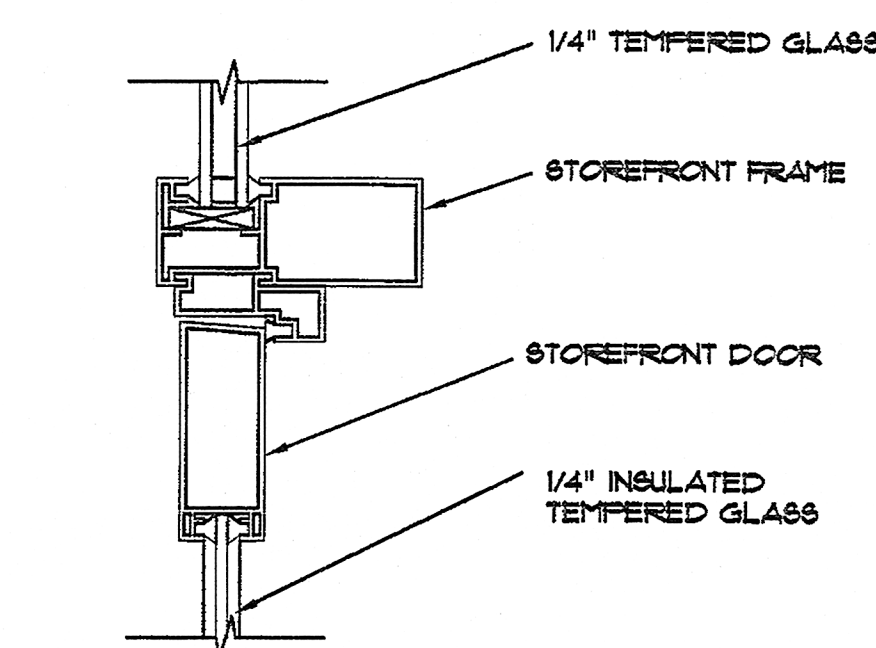
3 DOOR JAMB DETAIL SCALE: 3\"/>
