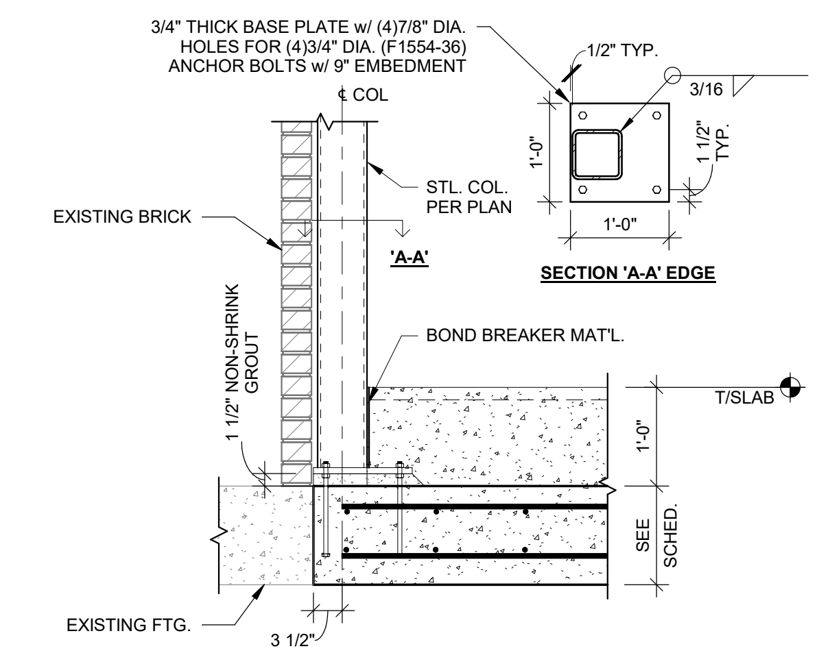
3 SECTION S301 SCALE: 3/4" = 1'-0"
