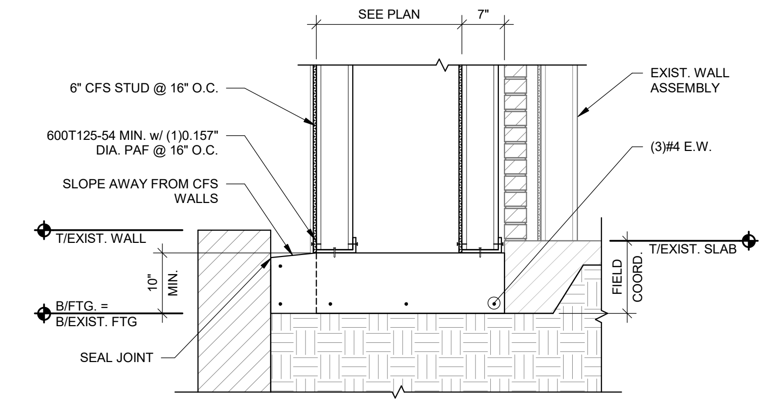
7 SECTION S301 SCALE: 3/4" = 1'-0"
